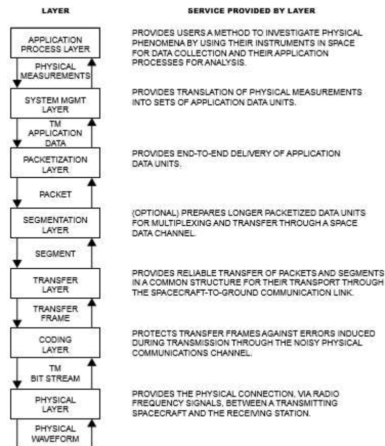
図1: テレメトリサービスの階層モデル
