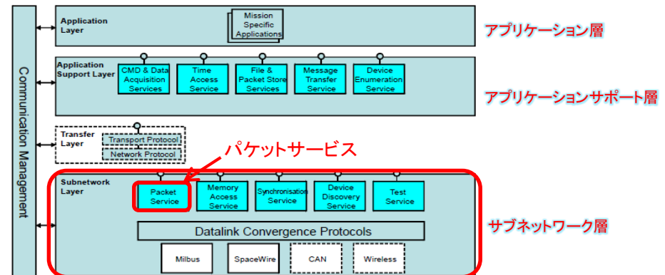
図1: サブネットワーク層のサービス関連図
