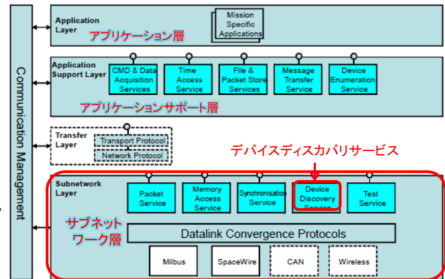
図1: サブネットワーク層のサービス関連図
