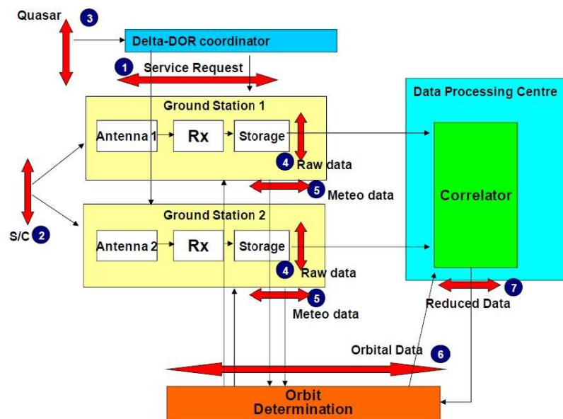
図4: Delta-DOR計測データフロー
