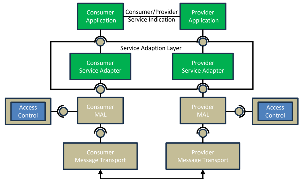
図1: MO の層構造
