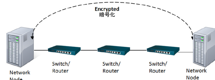
図2 エンドツーエンドのセキュリティサービス
