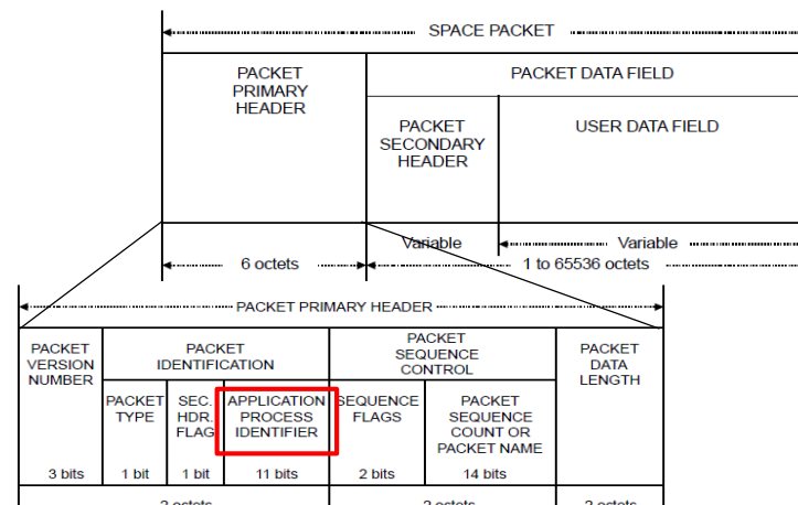
図2: スペースパケットの構造
