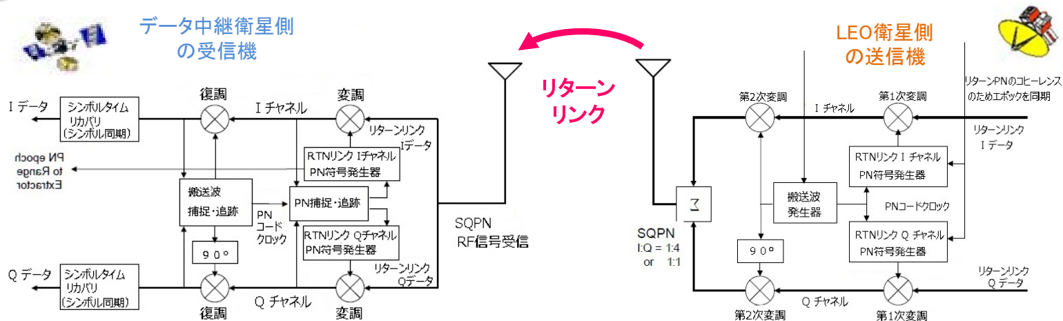
図2: 衛星ユーザー側からネットワーク側へのリターンリンク (例)
