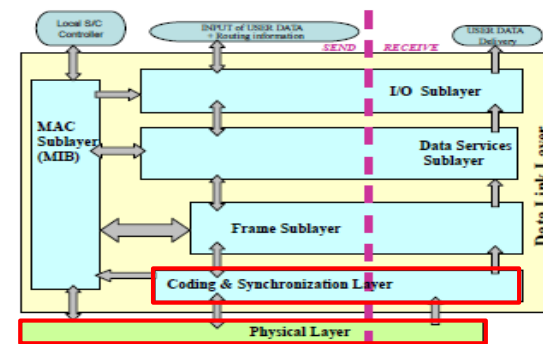
図2: 近傍領域通信-1のプロトコル概要
