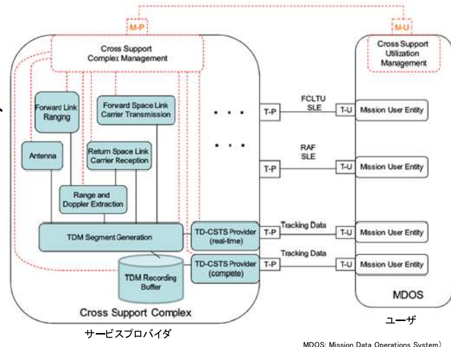
図1: CSTS追跡データサービス提供例
