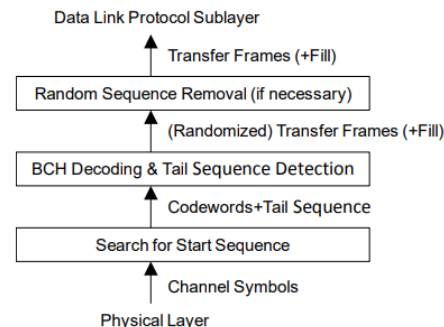
図3: 受信側の手順 (BCH復号化)
