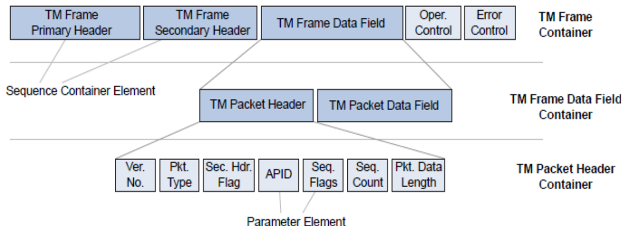
図1: XTCEによるデータベース交換のコンセプト
