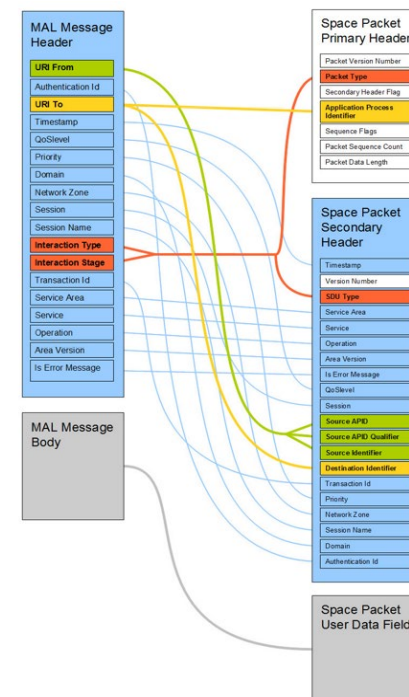
図4: MALメッセージ構造とスペースパケットのマッピング構造
