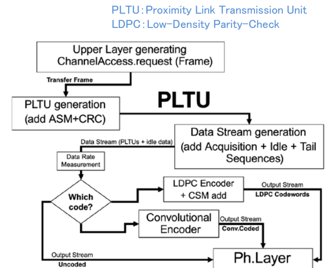
図2:コーディング&同期副層の処理フロー(送信側)
