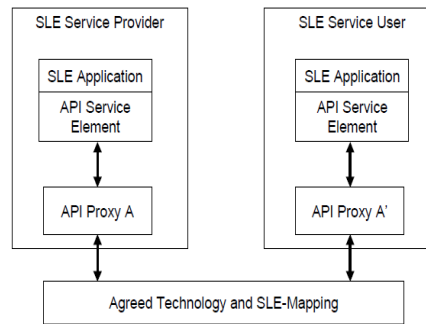
図7: SLEと他の技術のマッピングの共通化による相互運用性の実現
