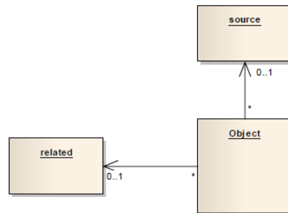
図2: COMの構造
