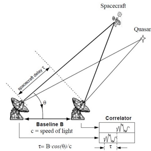
図1: DDOR観測
