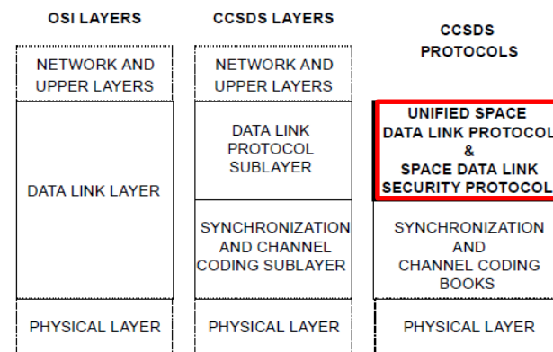
図1: USLP とOSI参照モデルの関係
