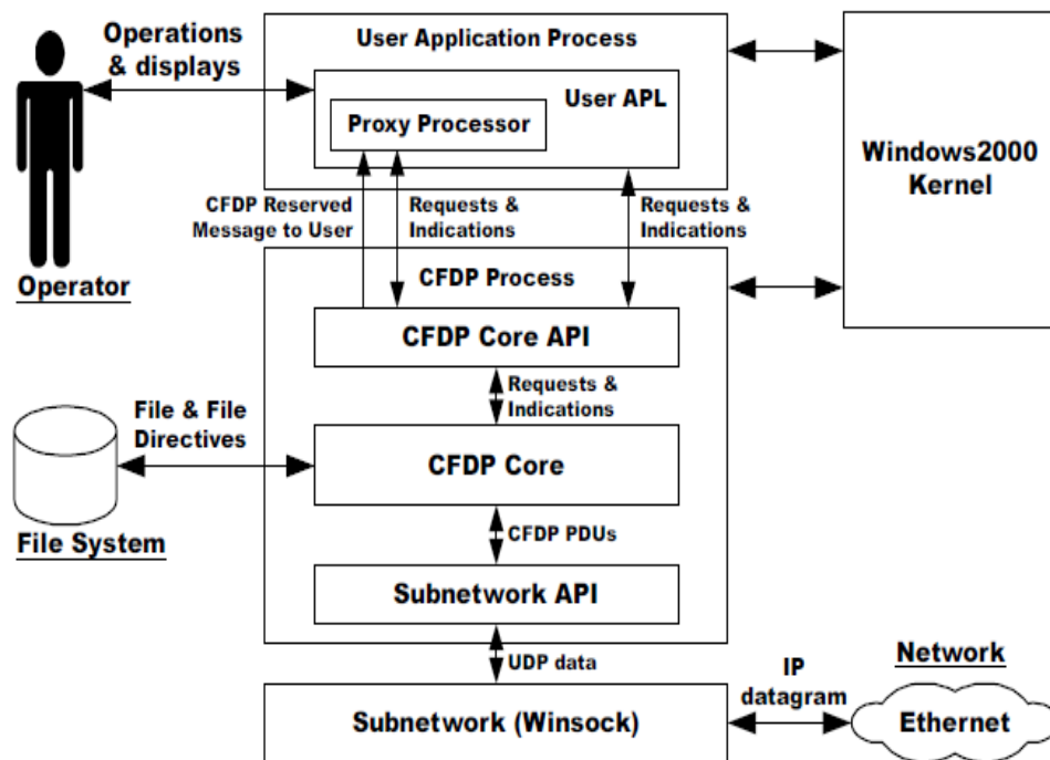
図3: JAXAにおけるCFDP実装アーキテクチャ
