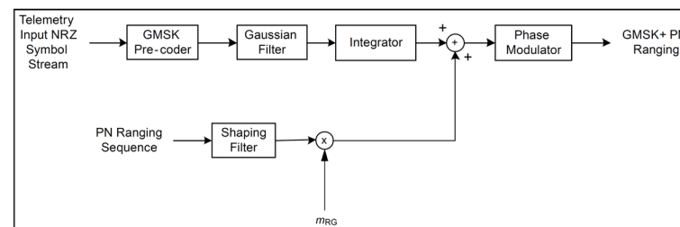
図1: GMSK+PN レンジング変調回路図(一例)
