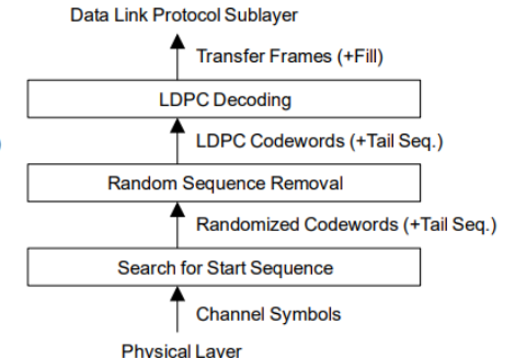
図4: 受信側の手順 (LDPC復号化)
