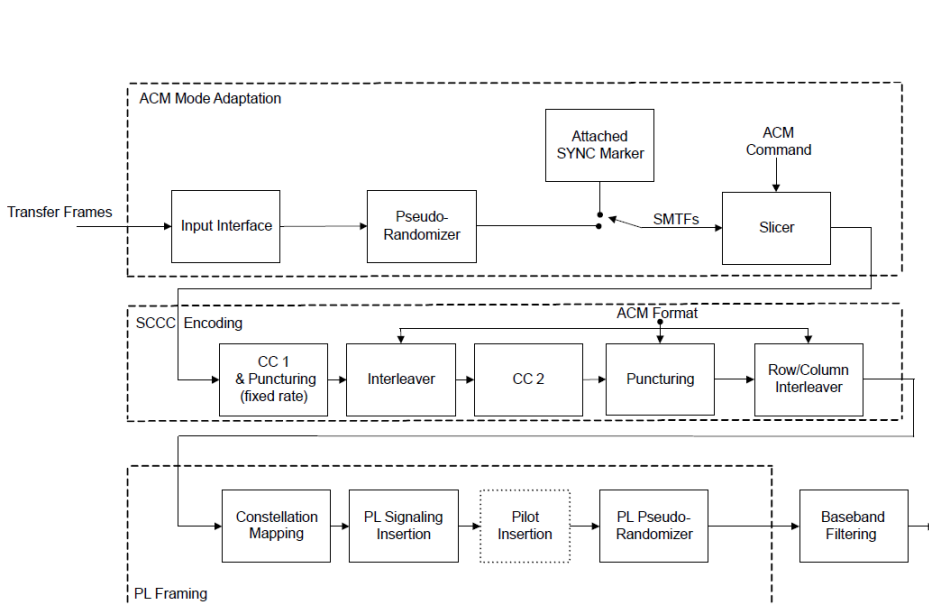
図1: 送信側の機能ブロック図
