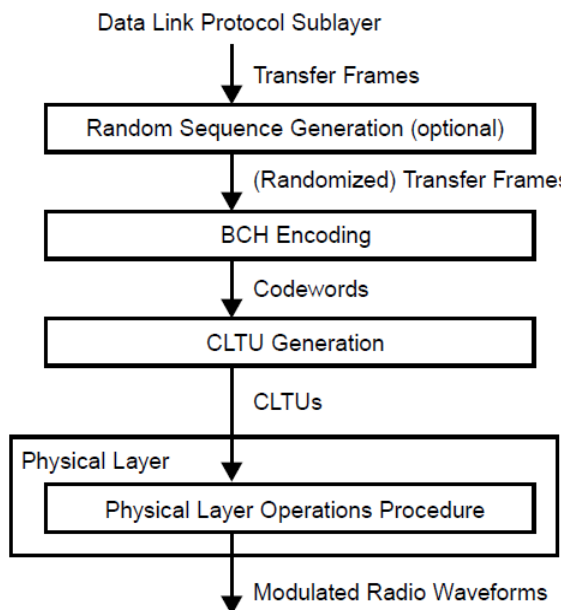
図1: BCHコーディングを使用した場合の送信側での内部構造
