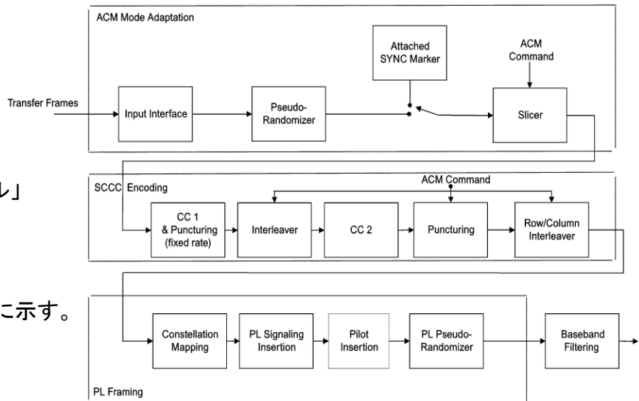
図1: 送信側の機能概念
