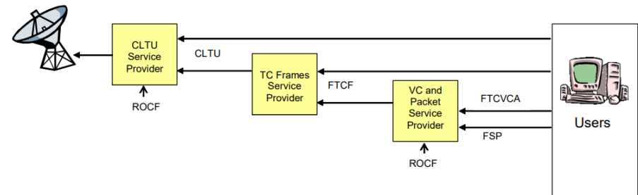
図2: Forward系SLE転送サービス概念
