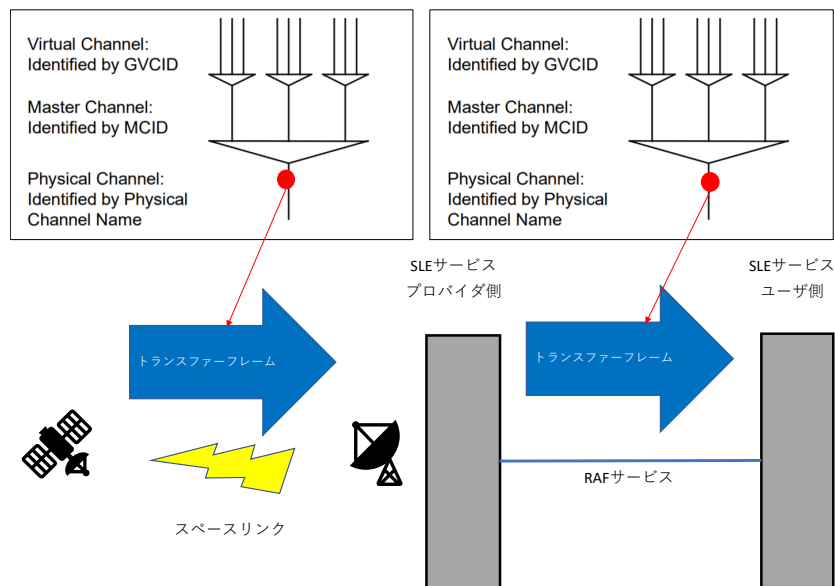
図3: RAFサービスのデータ転送
