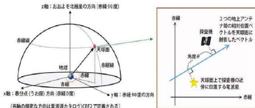
図1: Delta-DOR観測量の幾何学的意味
