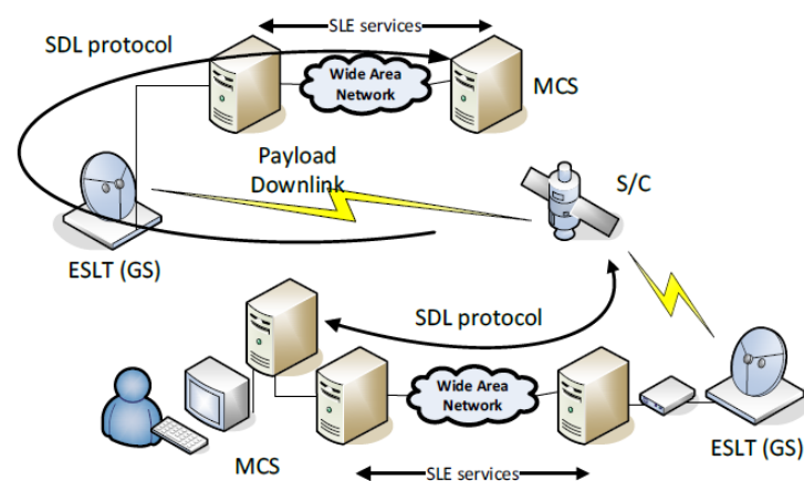
図1: ネットワークトポロジ例
