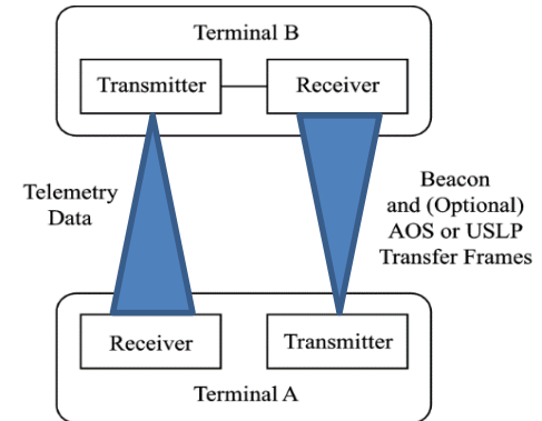
図1: トランスミッター(送信機)ーレーシーバー(受信機)間の光通信
