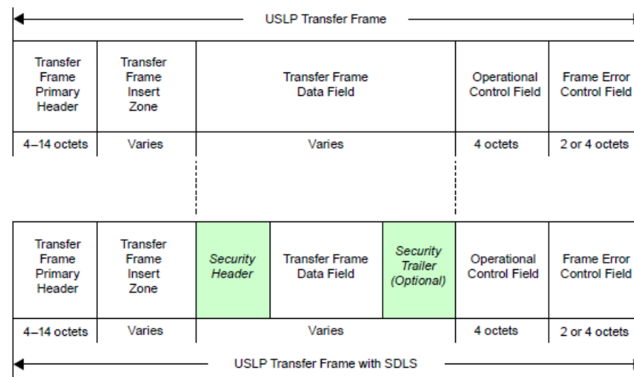
図2: USLPトランスファースフレームの構造
