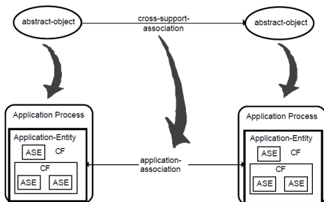
図6: ASDC モデルとアプリケーションサービスモデルのマッピング
