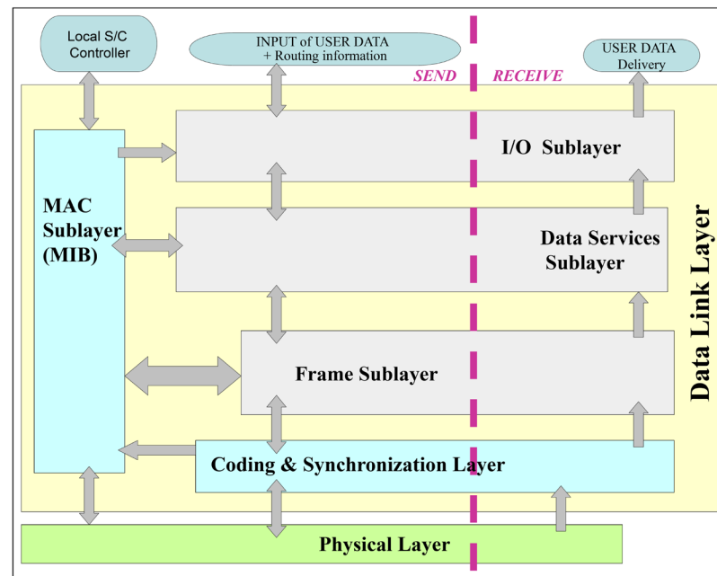
図1: 近傍領域通信-1のプロトコル概要
