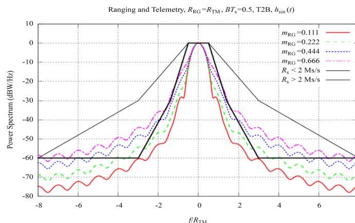
図2: GMSK/PNスペクトルプロット(一例) © 2022 宇宙航空研究開発機構(JAXA)
