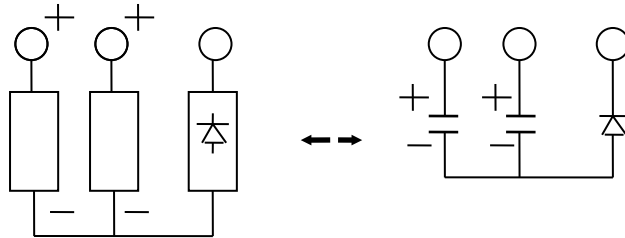
回路図
