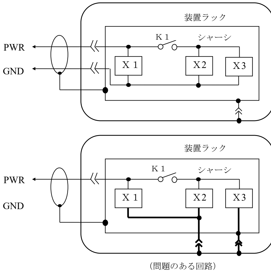
図3.28-5 スニーク回路の例
