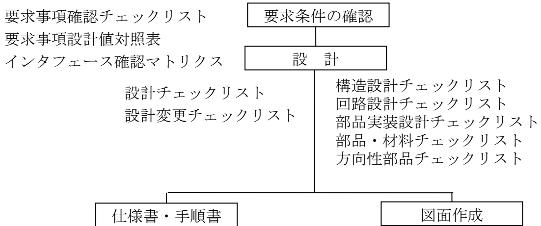
図3.32-1 チェックリストの体系の例
