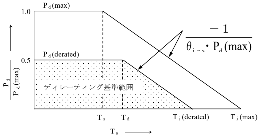
付図ー１ 電力のディレーティング値VS接合部温度ディレーティング値 (ヒートシンクなしの場合)
