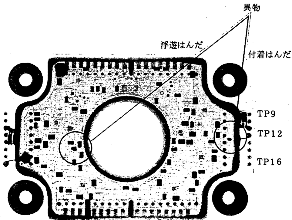
写真3. 38-7 ハイブリッドICの異物混入
