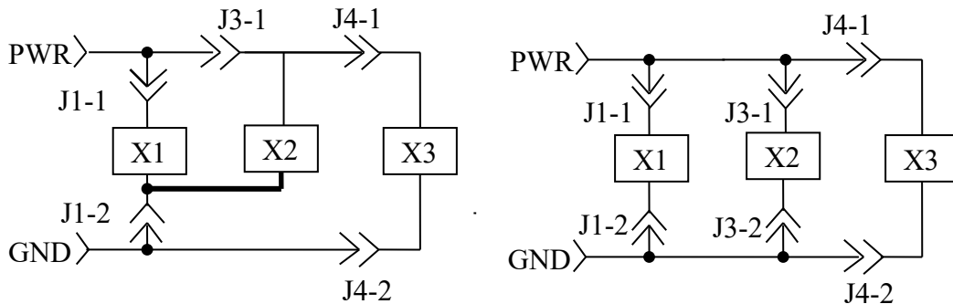
図3. 28-10 スニーク回路の例
