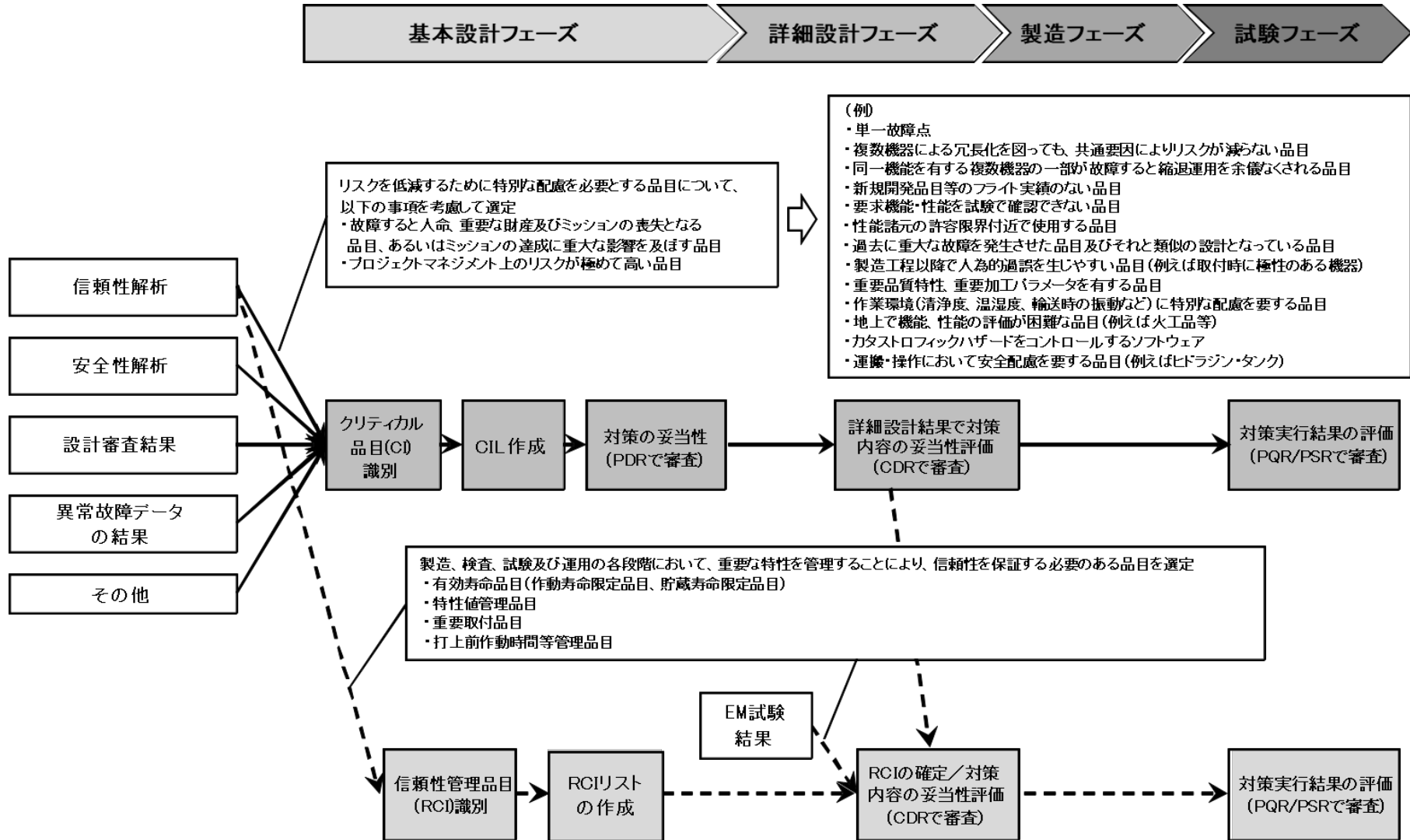
図3.42-2 特別な管理を要する品目の識別・管理フロー
