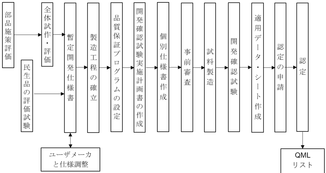
図3.54-3 JAXA-QTS-2000による共通部品の開発／認定フロー
