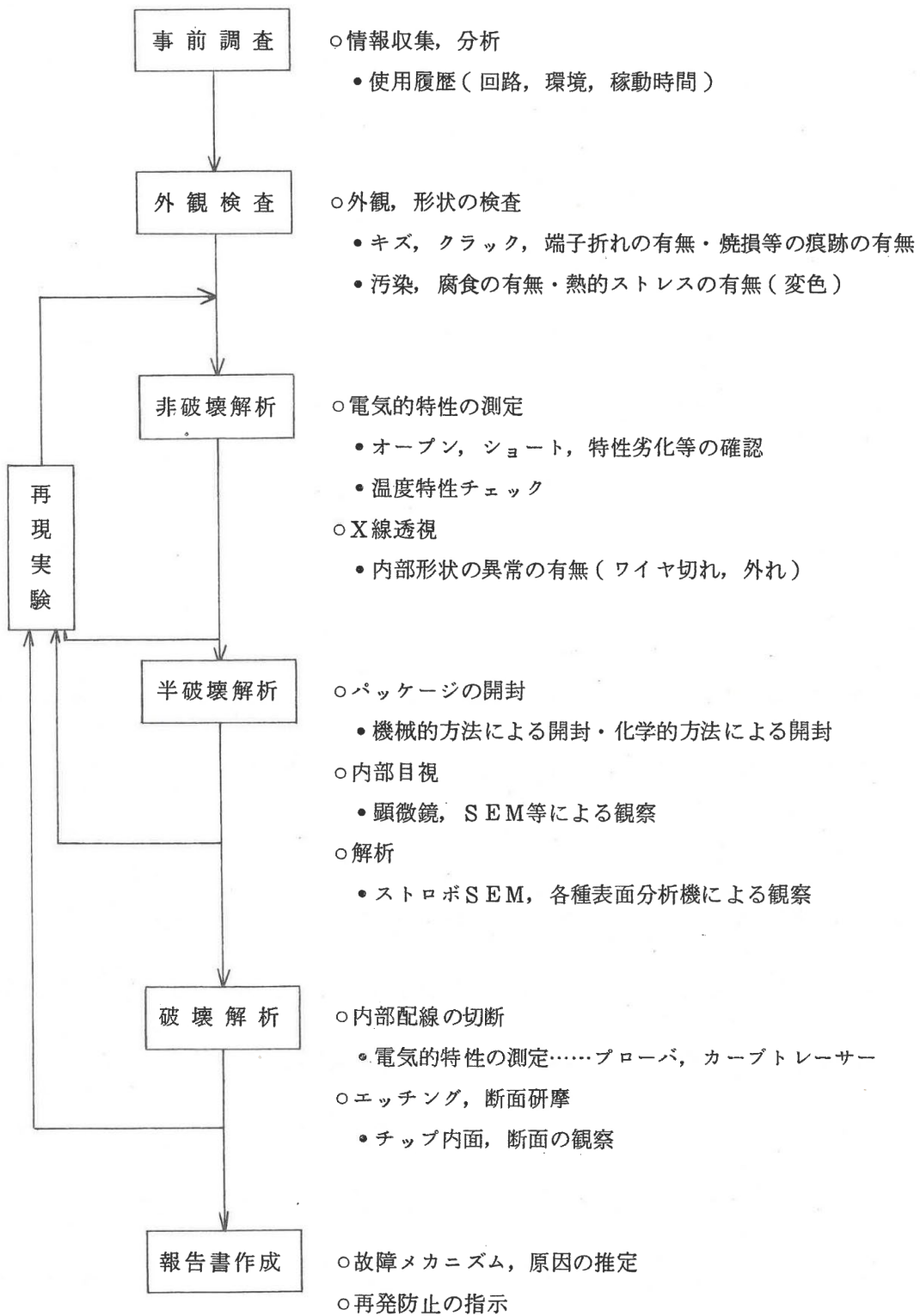
図3.38-2 半導体デバイスの故障解析手順(例) 3)
