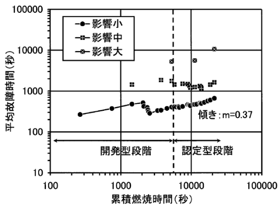
図3.12-7 LE-7Aエンジンの信頼度成長 5)
