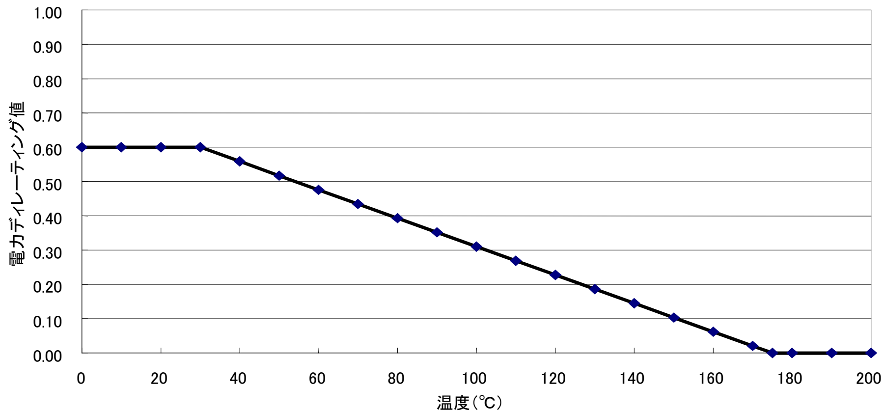
図3.15-2 抵抗器 (RWR) のデレーティング基準曲線
