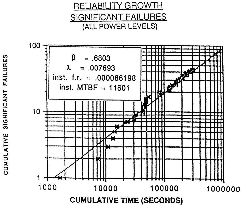
図3.12-9 SSME信頼度成長 (重大な故障) 6)
