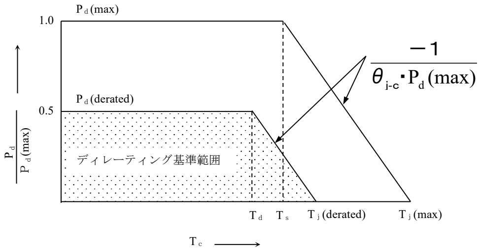
付図-2 電力のディレーティング値VS接合部温度ディレーティング値 (ヒートシンク付の場合)
