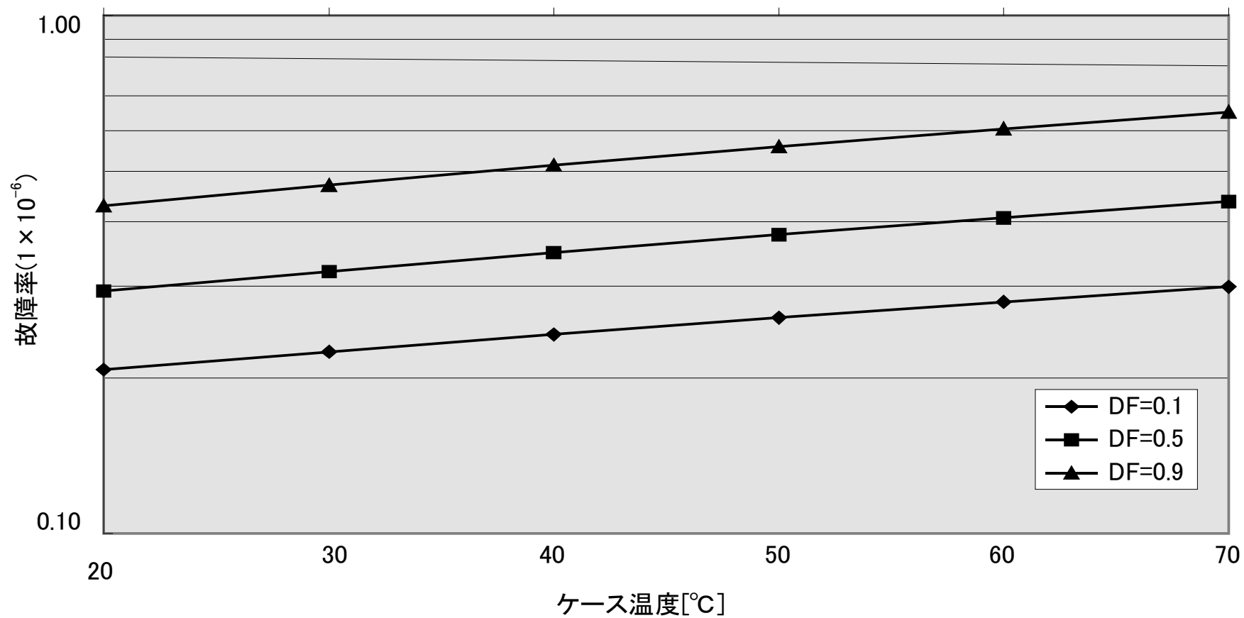
図3.15-1 DF値と故障率の関係
