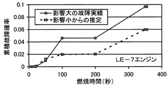
図3.12-6 故障分布法による信頼度の推定 5)
