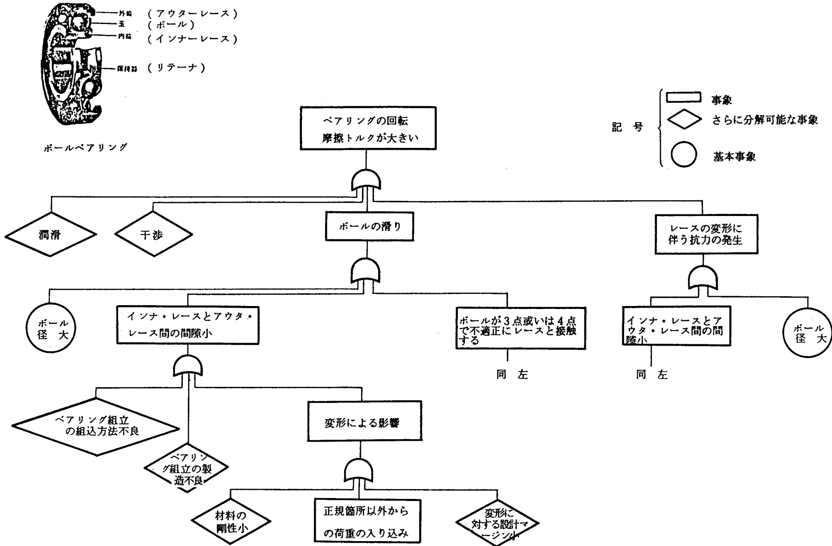
図3. 25-2 ベアリングの不具合に関するFTA
