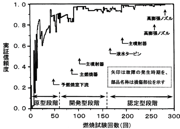
図3.12-4 LE-7エンジンの信頼度推定(従来法) 5)
