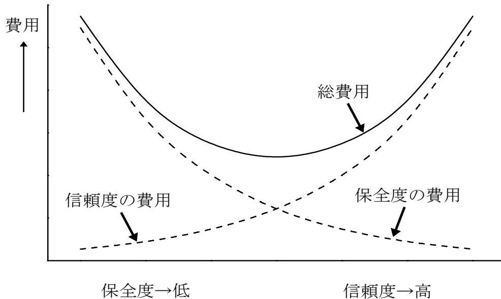
付図 3-4 信頼度と保全度の最適化
