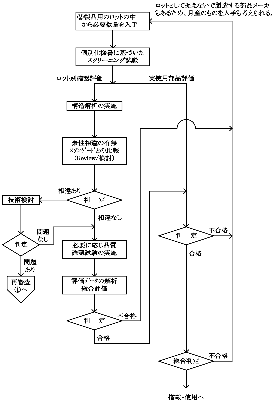
図3.52-2 民生部品適用判定／搭載判定評価詳細フロー (2/2)
