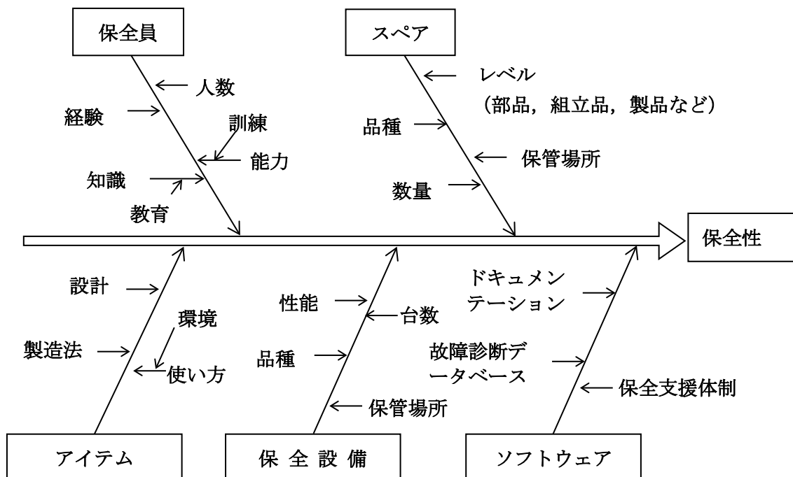
付図 3-3 保全性支援能力を決める要因
