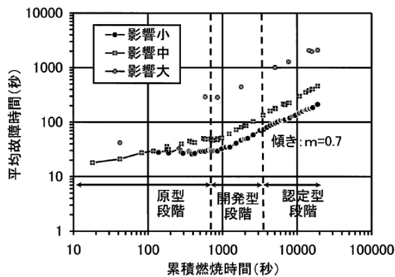
図3.12-5 LE-7エンジンの信頼度成長 5)
