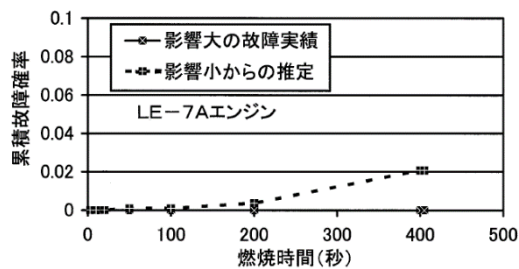
図3.12-8 故障分布法による信頼度の推定 5)
