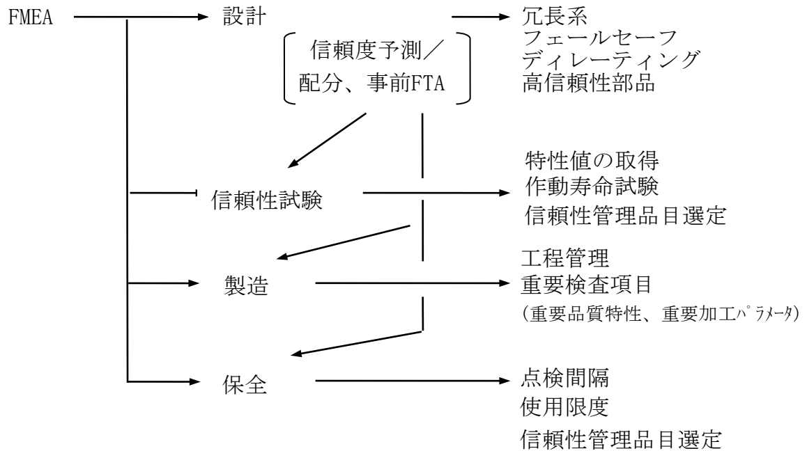
図3.16-1 FMEA活用例
