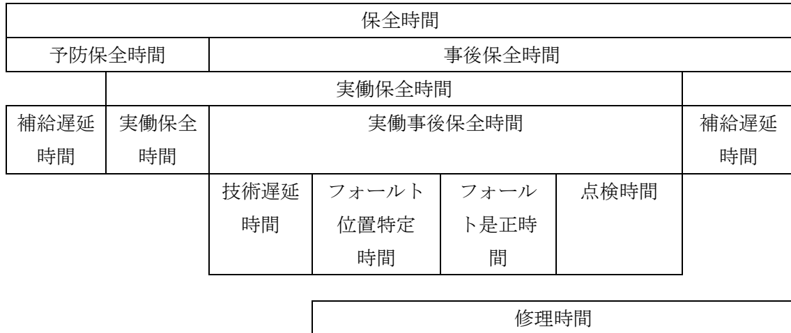
付図 3-2 保全時間のダイアグラム
