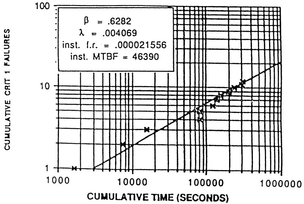
図3.12-10 SSME信頼度成長（クリティカリティ1の故障） 6)
