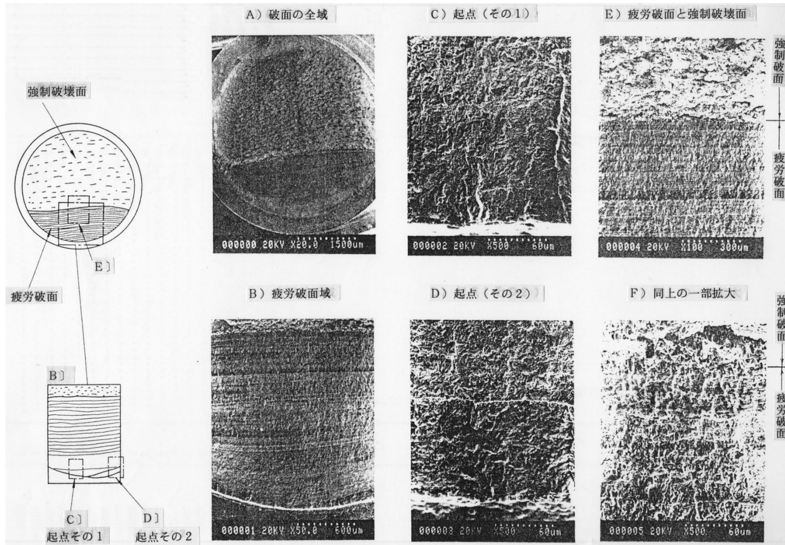
写真3.38-2 電子顕微鏡によるNo.1取付ボルトの破面観察結果
