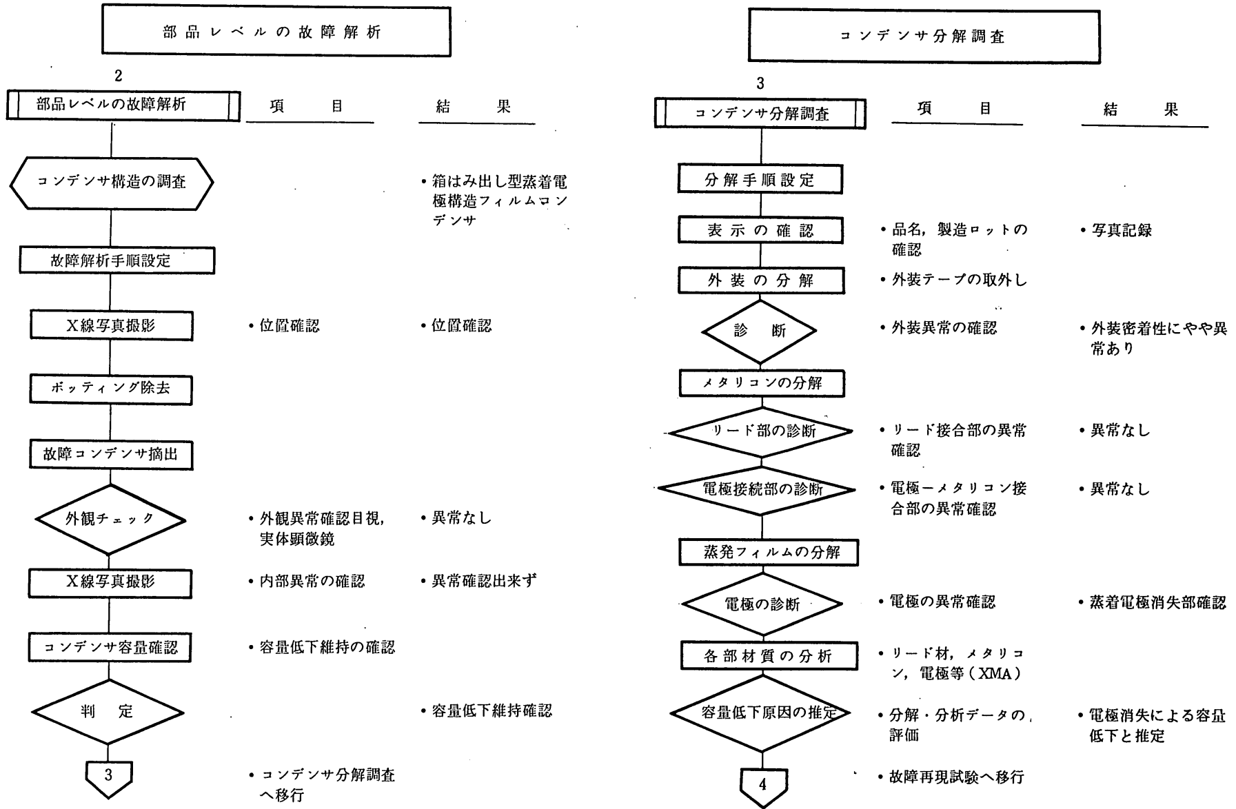
図3. 38-3 機器レベルから部品（コンデンサ）レベルまでの故障解析手順（例）（2/2）
