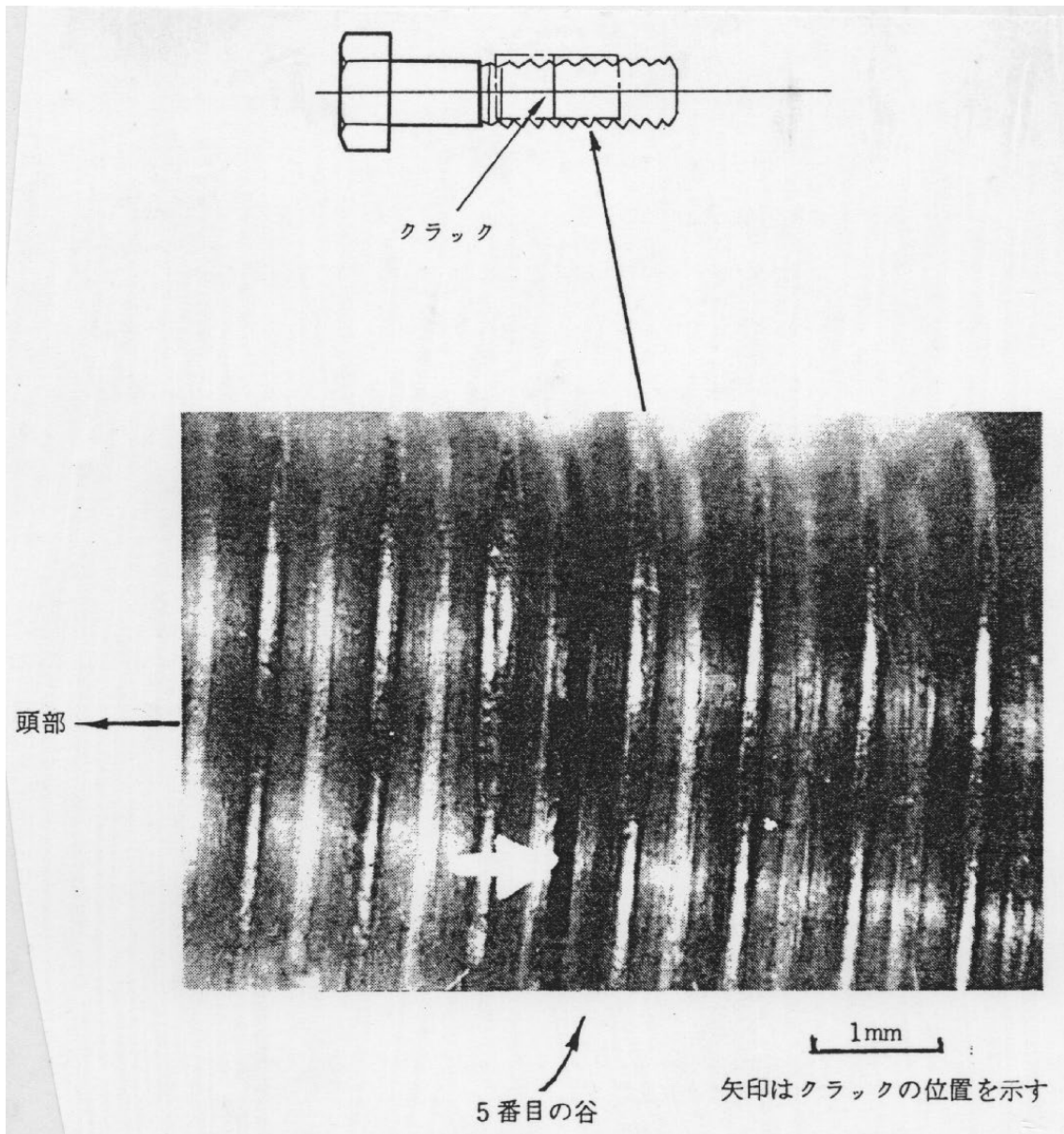
写真3.38-1 No.1ボルトのクラック発生状況
