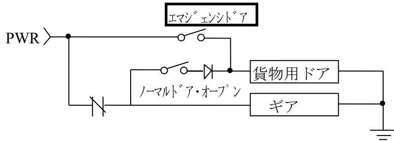
図3. 28-9 スニーク表示の例
