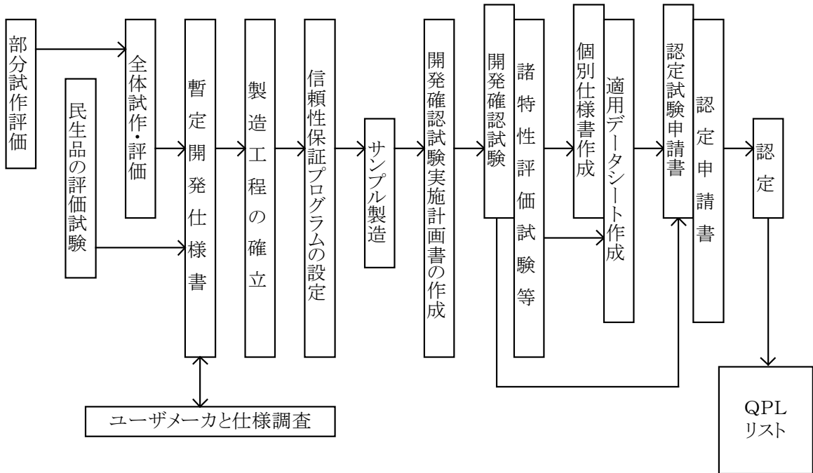
図3.54-2 NASDA-QTS-38100による共通部品の開発／認定フロー
