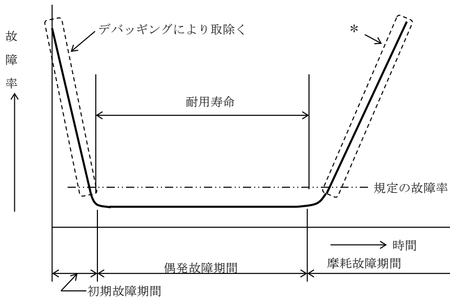
図3.12-1 バスタブ曲線(Bath-Tub Curve)
