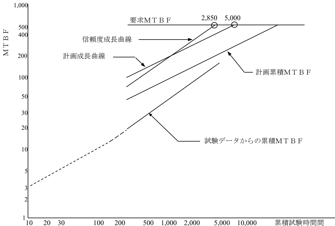
図3.12-2 デュアンの信頼性成長モデル 3)
