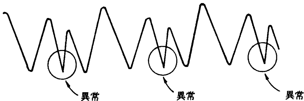
図3.37-4 ジャイロ出力波形異常例(2)
