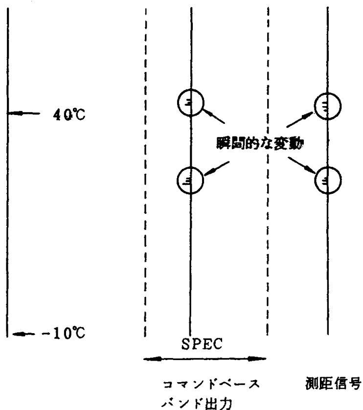
図3.37-2 受信機出力異常
