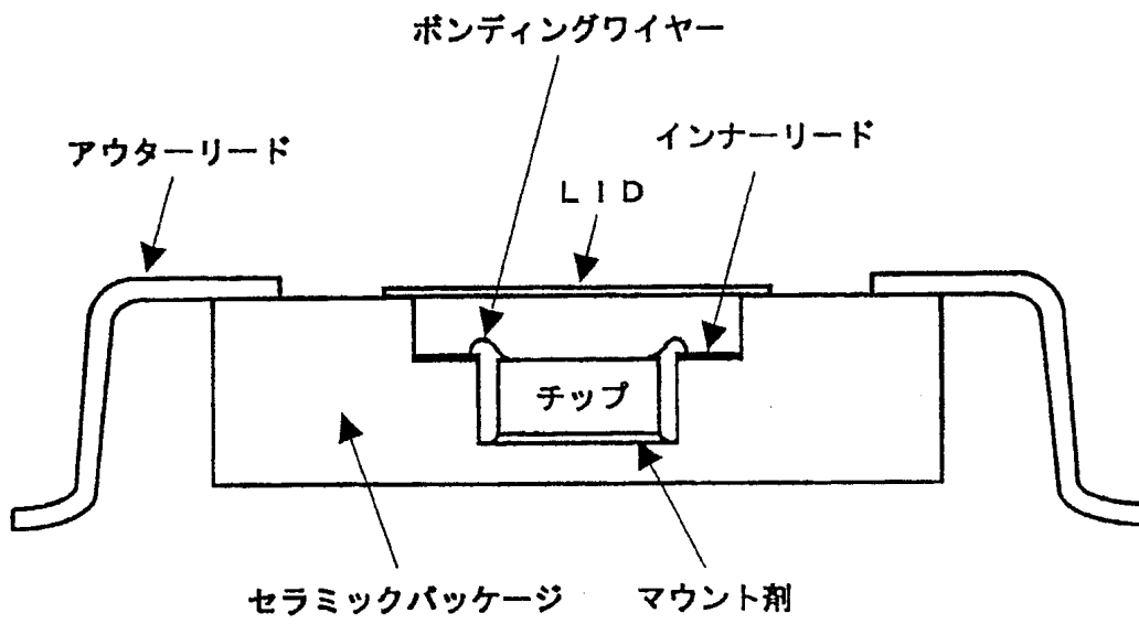
図3.37-7 MPU構造概略図
