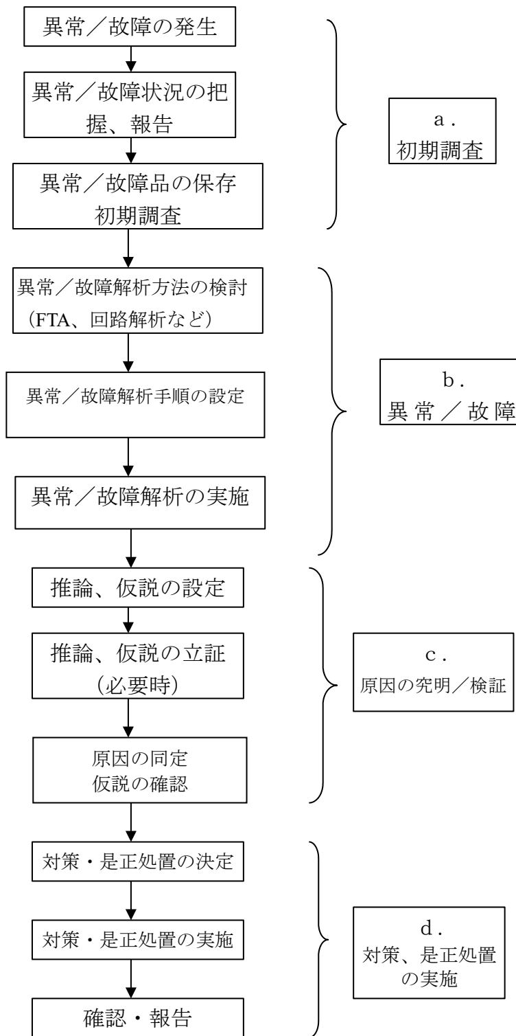
図 3.38-1 異常 / 故障管理フロー
