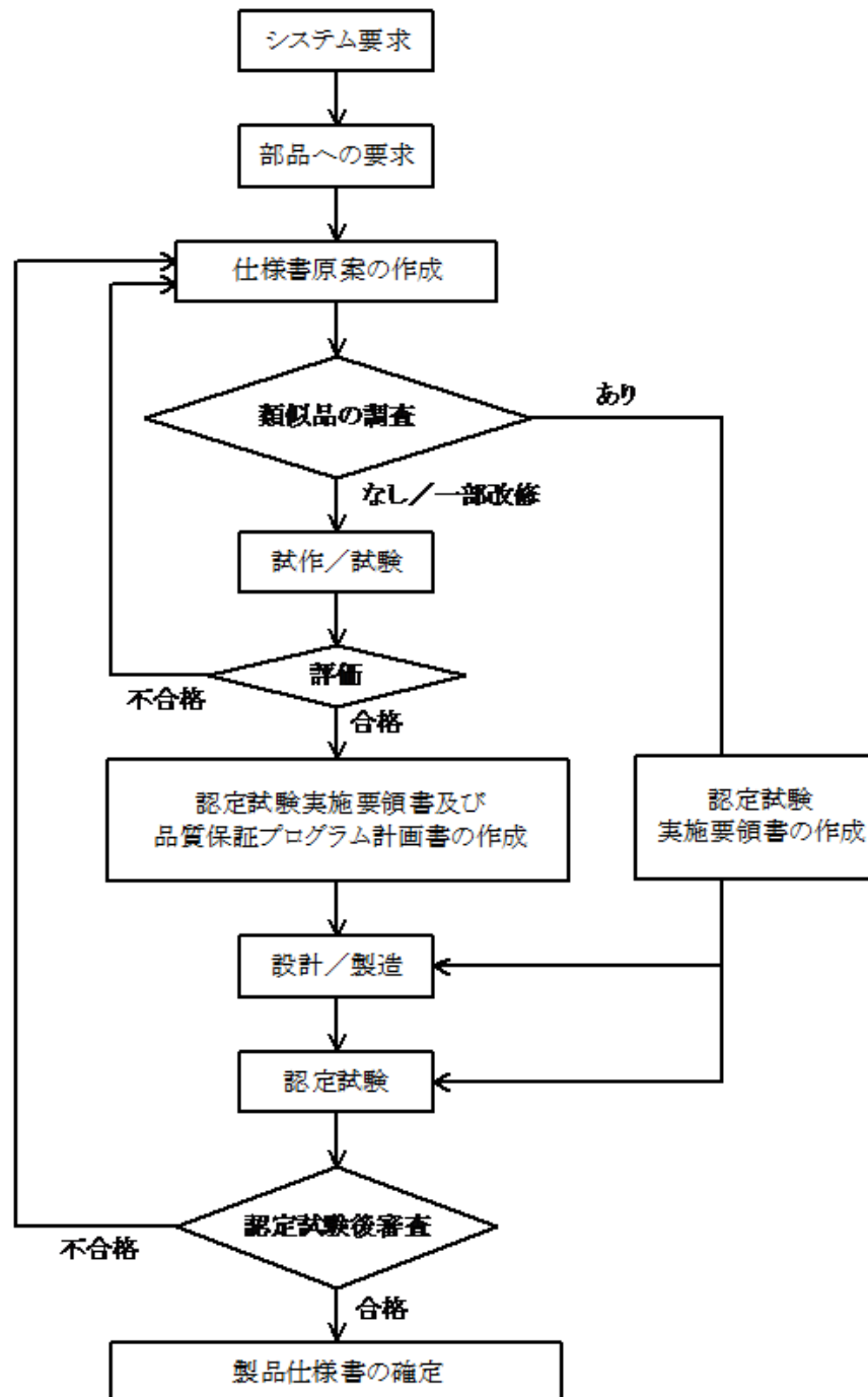
図3.54-1 プロジェクト認定のフロー
