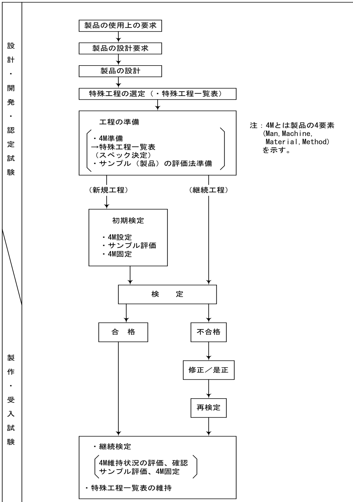
図3.57-2 特殊工程全体フロー
