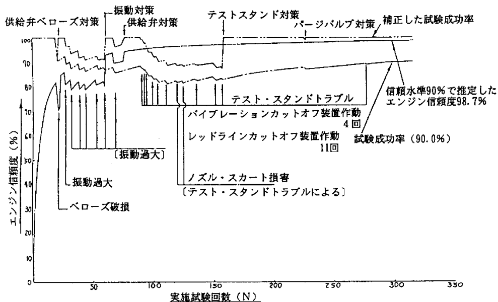
図 3.12-3 ロケット用エンジンの信頼度 4)
