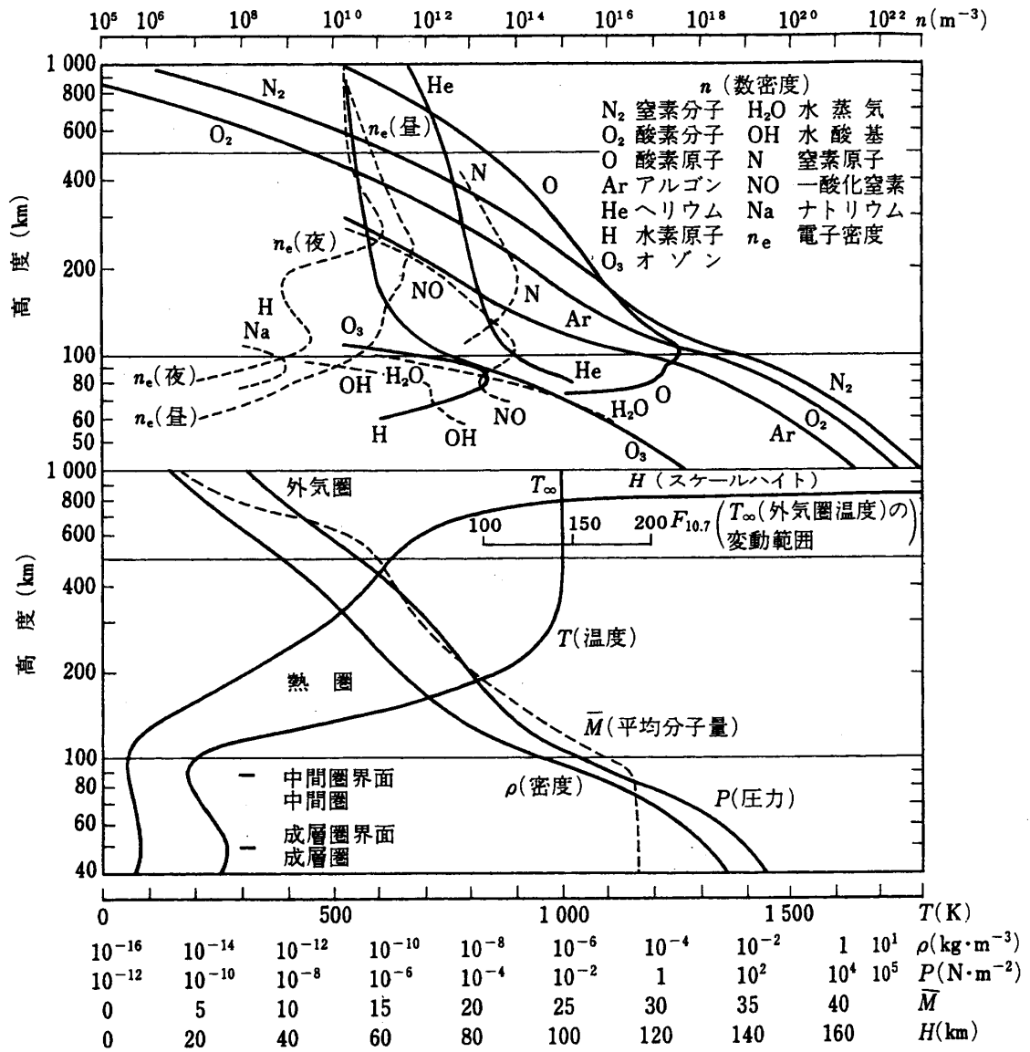
図3.3-1 地球高層大気物性の高さ分布
