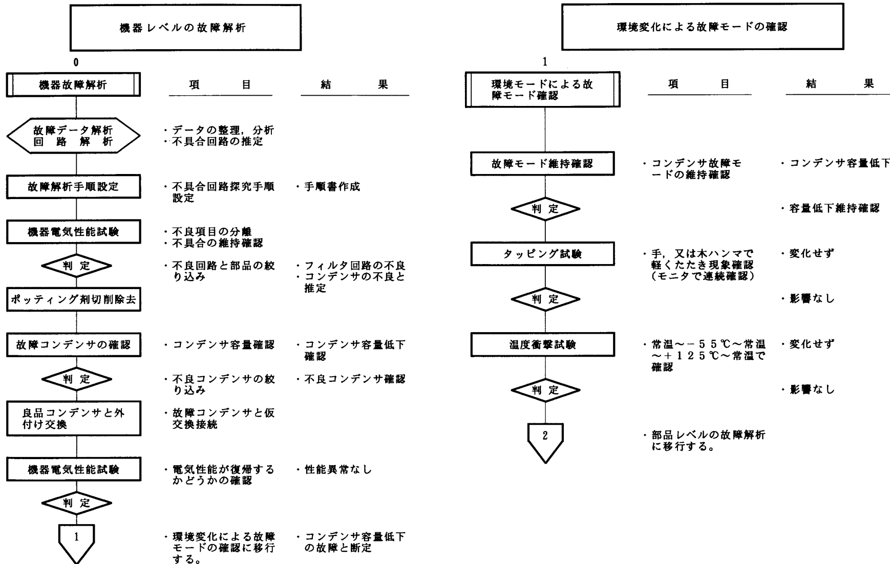
図3.38-3 機器レベルから部品（コンデンサ）レベルまでの故障解析手順（例）（1/2）
