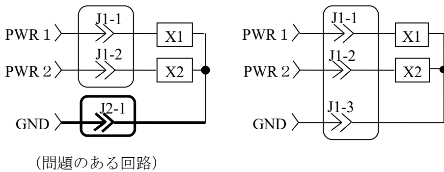
図3.28-12 スニーク回路の例
