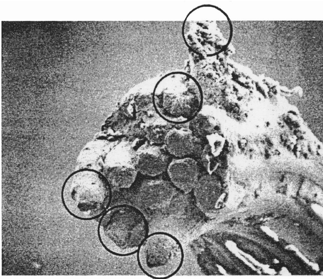
写真3.38-3 より線破断のSEM像
