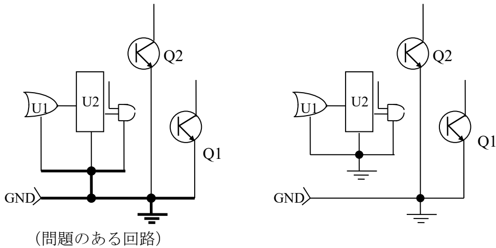
図3. 28-14 スニーク回路の例
