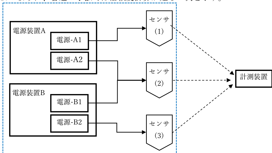
図3.12-13 通常の手法では信頼度計算が困難な例
