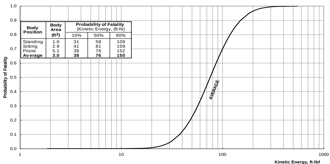
図3.3-2：落下物のエネルギーと致命率の関係（出典：参考文献(5)）
