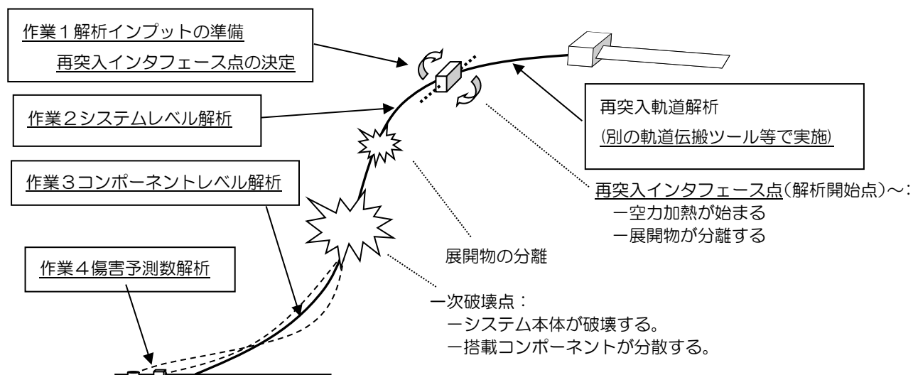
図2.2-1 落下経路に沿ったフェーズの概念
