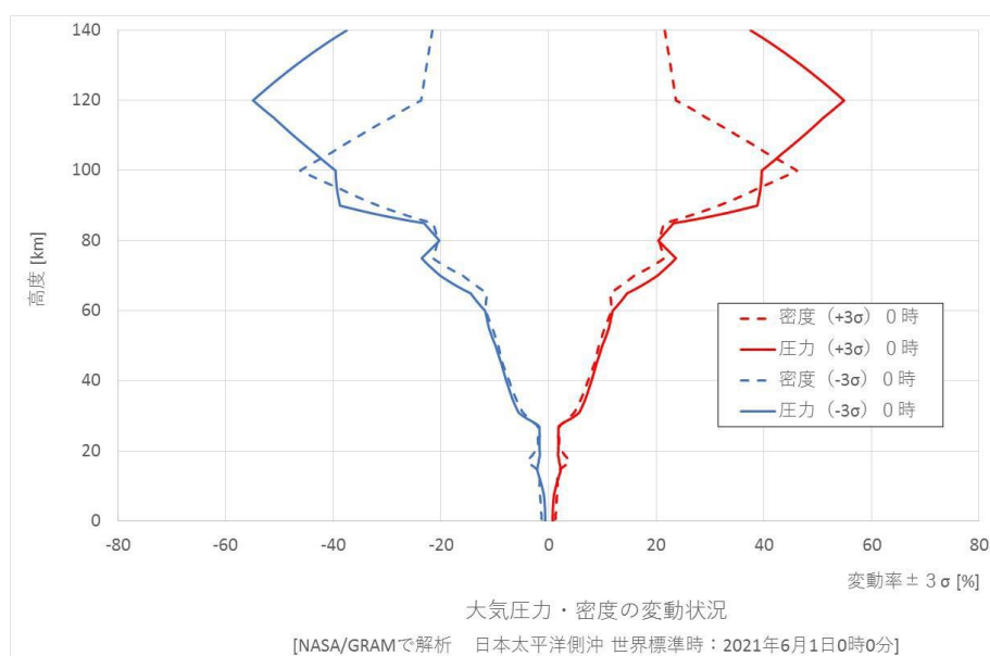
図3.1-2 NASA- Earth Global Reference Atmospheric Modelによる大気圧力・密度の変動例
